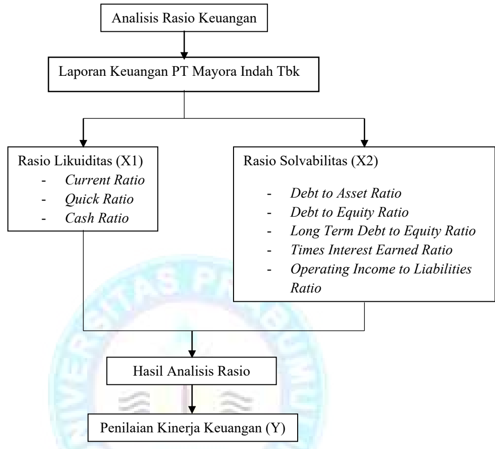
Gambar 2.1 Kerangka Pemikiran
